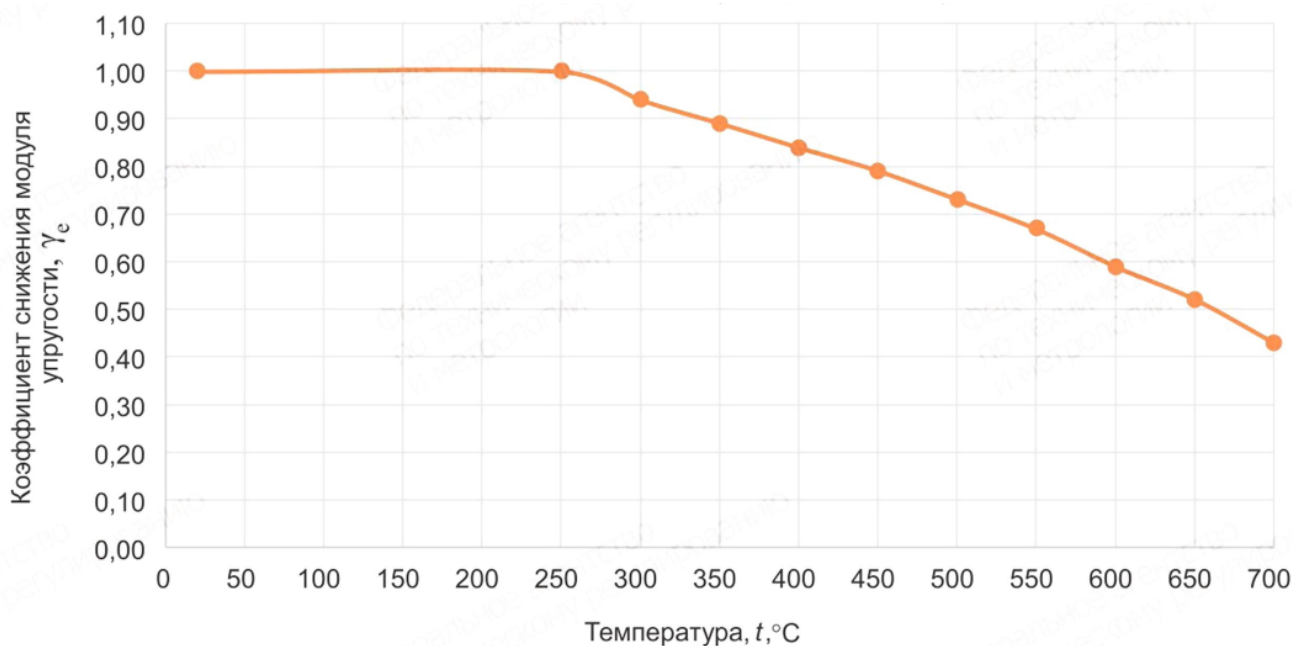
Рисунок Б.1 - Температурный коэффициент снижения модуля упругости ( \gamma_e ) стали обычной прочности (С235, С245, С255)
