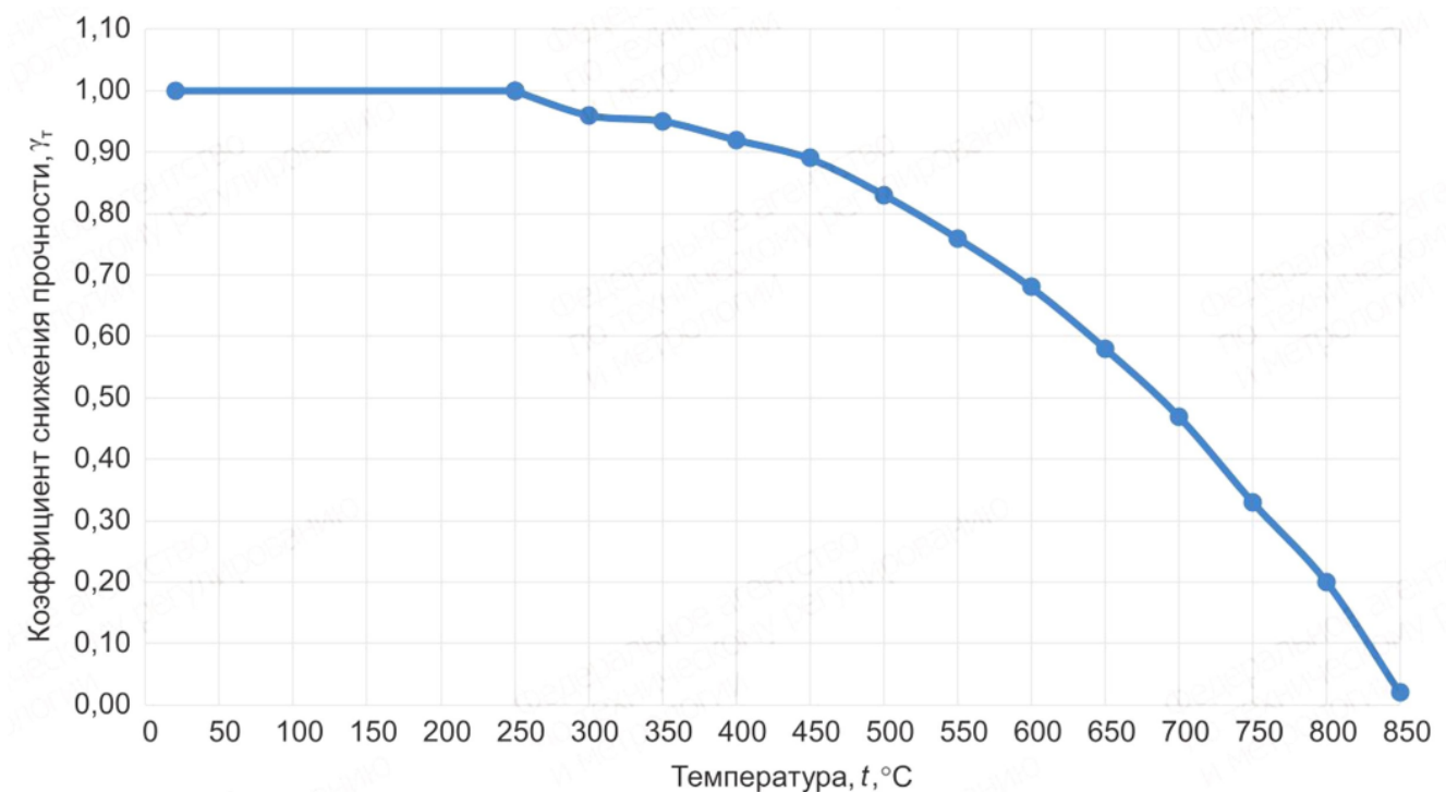
Рисунок Б.8 - Температурный коэффициент снижения прочности ( \gamma_T ) огнестойкой стали (С355П, С390П)
