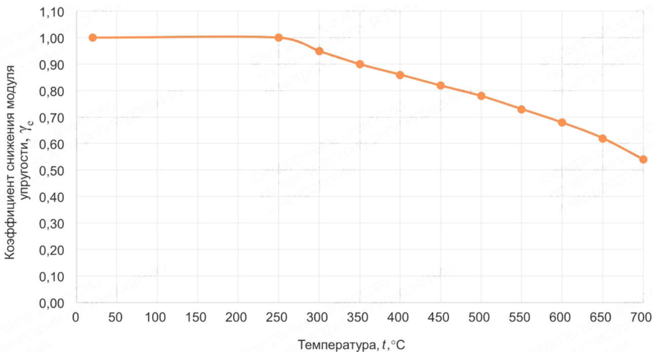
Рисунок Б.3 - Температурный коэффициент снижения модуля упругости ( \gamma_e ) стали высокой прочности (С390, С390-1, С440, С550, С590)
