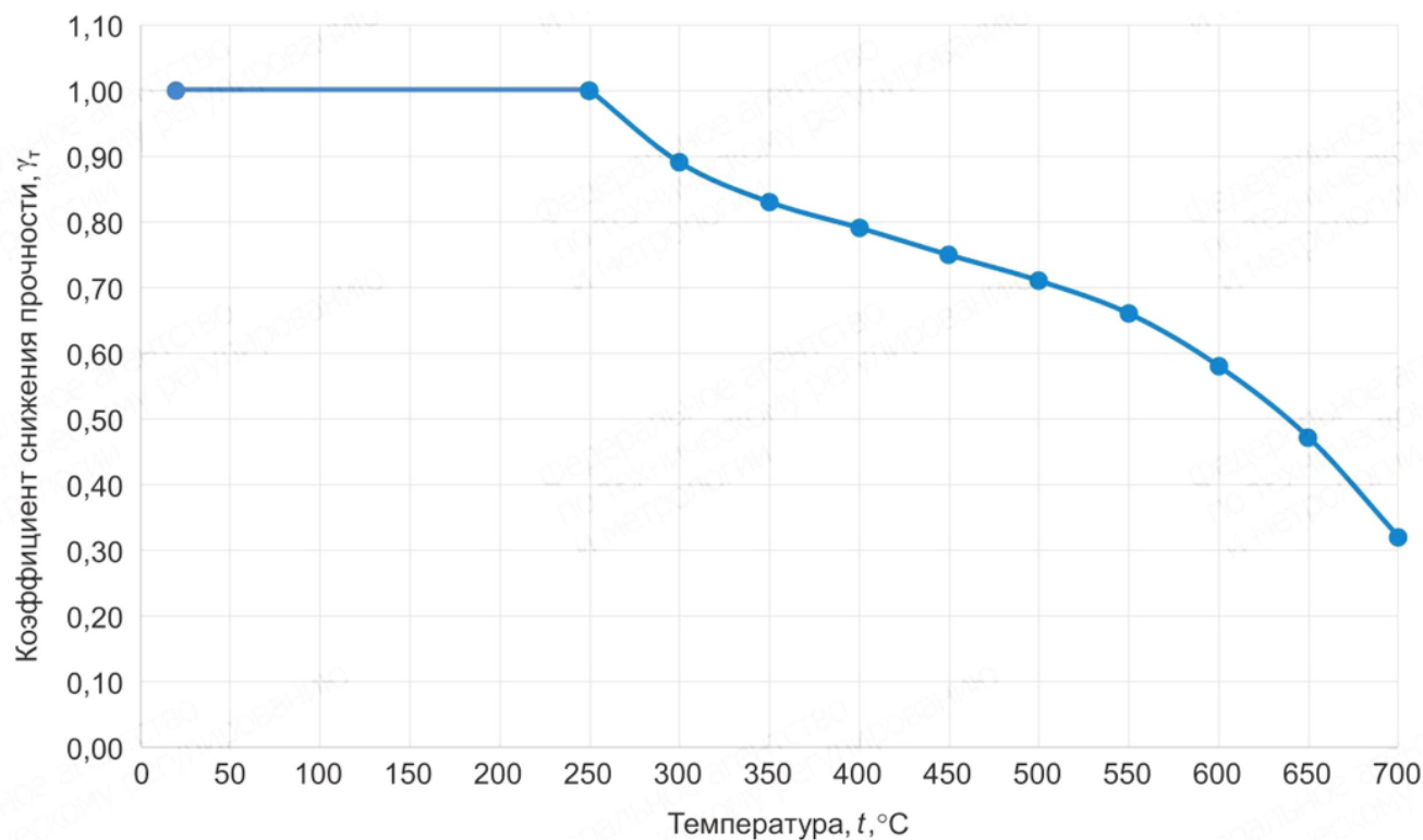
Рисунок Б.7 - Температурный коэффициент снижения прочности ( \gamma_T ) стали высокой прочности
