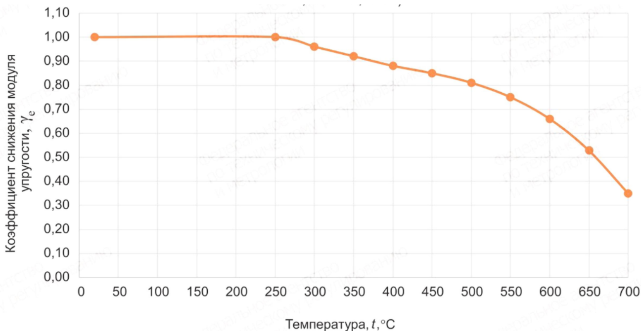
Рисунок Б.2 - Температурный коэффициент снижения модуля упругости ( \gamma_e ) стали повышенной прочности (С345, С345К, С355, С355-1, С355-К, С375)
