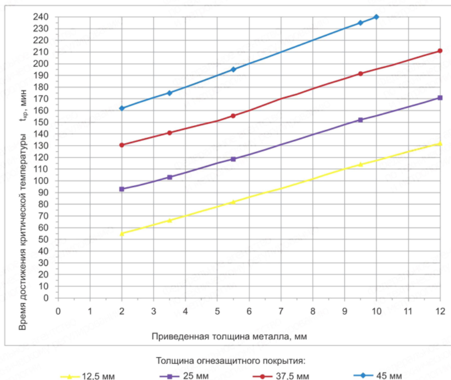
Рисунок 3 - Пример номограммы нагрева стальных конструкций с огнезащитным покрытием при стандартном температурном режиме пожара до t_{кр} = 600^{\circ}\text{C}
