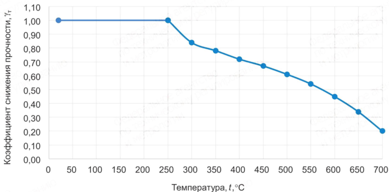
Рисунок Б.5 - Температурный коэффициент снижения прочности ( \gamma_T ) стали обычной прочности С235, С245, С255
