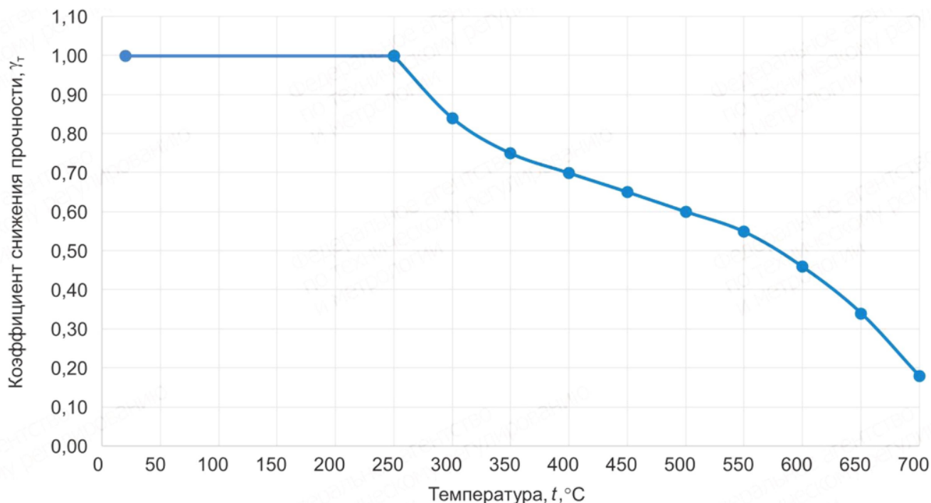
Рисунок Б.6 - Температурный коэффициент снижения прочности ( \gamma_T ) стали повышенной прочности (С345, С345К, С355, С355-1, С355-К, С375)
