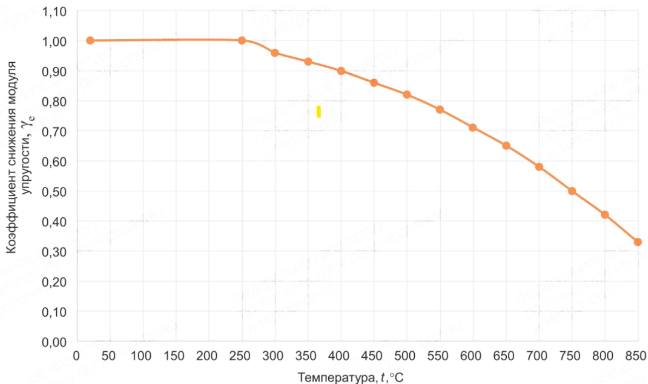
Рисунок Б.4 - Температурный коэффициент снижения модуля упругости ( \gamma_\epsilon ) огнестойких сталей (С355П, С390П)
